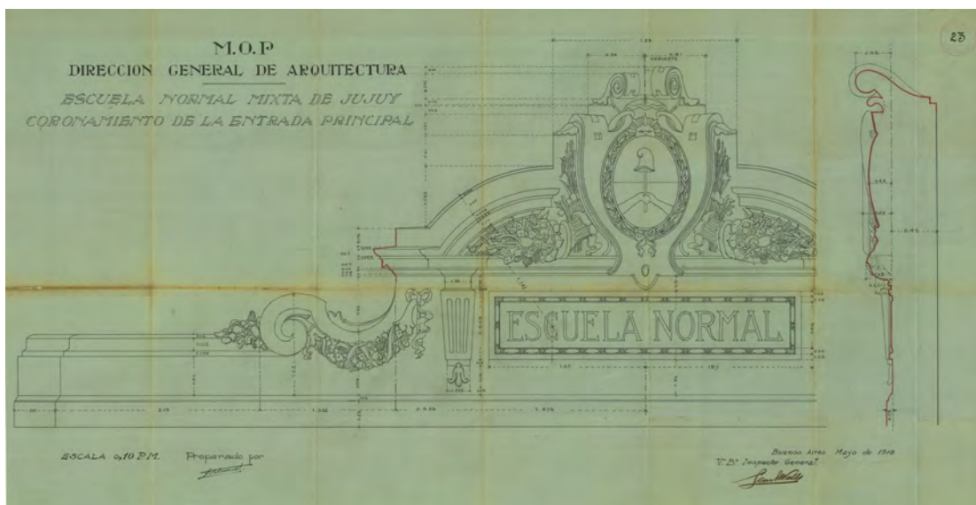
Figura 9. René Villeminot. Escuela Normal Mixta de San Salvador de Jujuy, (1918). Detalle del escudo en el cuerpo central de la fachada principal. Sección y vista. Documento perteneciente al archivo del Centro de Documentación e Investigación de la Arquitectura Pública –CeDIAP– del Ministerio de Economía y Finanzas Públicas.
